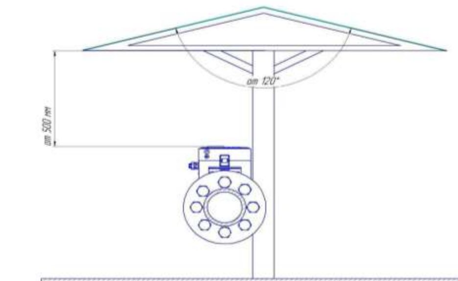
Рисунок 13 - Установка расходомера UMG под навесом.
