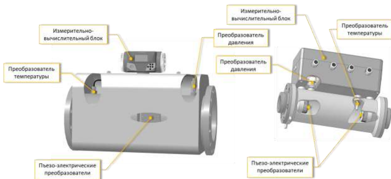
Рисунок 5 – Конструктивное устройство расходомера UMG
