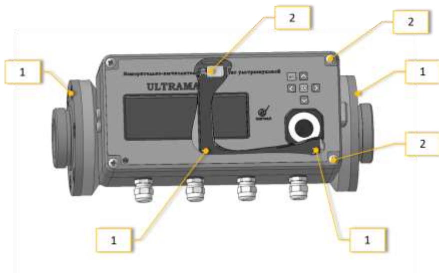
Рисунок 9 –Пломбировка варианта расходомера UMG с базовым ИВБ, резьбовым соединением и аксиальным расположением ПЭП
