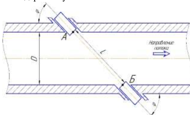
Рисунок 3 – Схема одноканального УЗР с ПЭП
