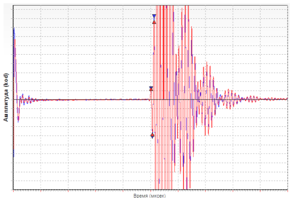
Рисунок 4 - Типовой вид осциллограммы измерительного сигнала
